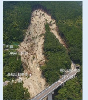
大豊町立川千本で発生した山腹崩壊（平成30年7月撮影）
